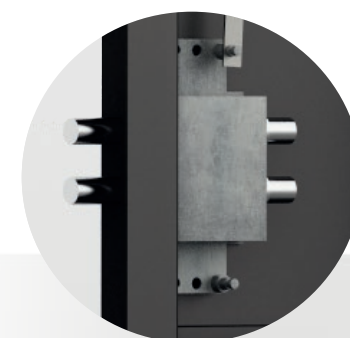
Deviatore doppio a slitta inferiore
